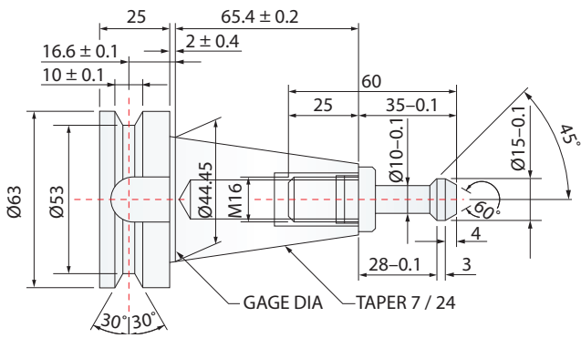
BT40
