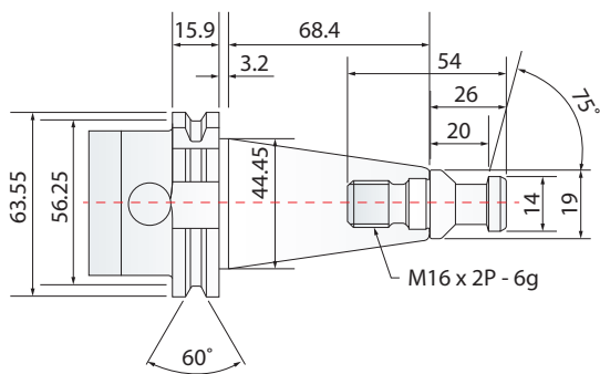
DIN40
