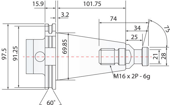
DIN50
