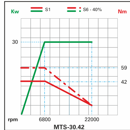
Motore AC sincro • Synchronous-motor Synchron-Motor • Moteur synchrone
