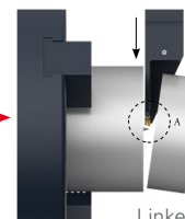
Abstechen ohne Ansatz
