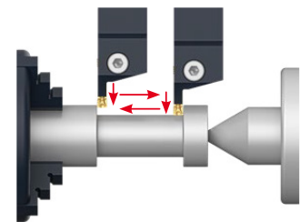
Einstechen / Längsdrehen zweiseitig
