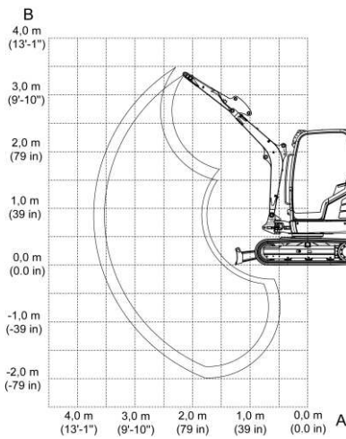
Abb. 1: Hubkrafttabelle Oberwagen nicht gekippt
