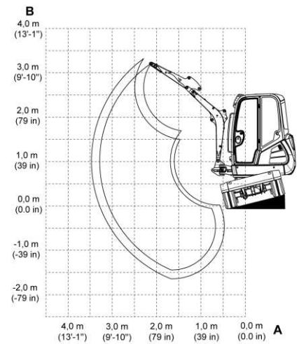
Abb. 3: Hubkrafttabelle – Oberwagen gekippt, Armsystem bergauf (Hangneigung 15°)
