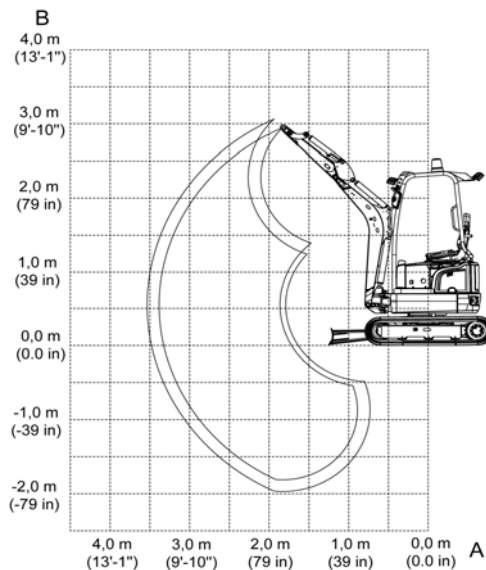
Abb. 1: Hubkrafttabelle EZ17
