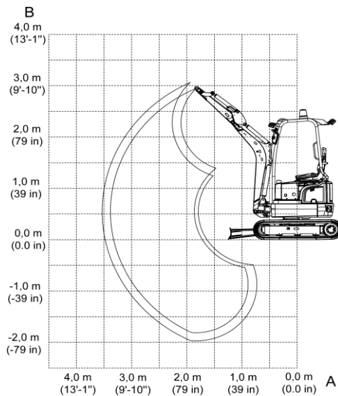
Abb. 1: Hubkrafttabelle EZ17e
