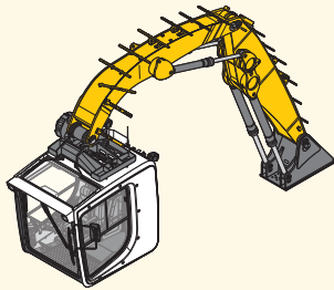
Hydraulische Kabinenerhöhung
