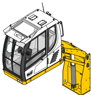
Hydraulische Kabinenerhöhung
