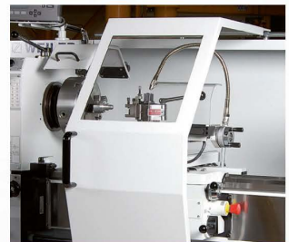
Verfahrbare, umfassende Spänespritzschutzhäube mit Sichtfenster
